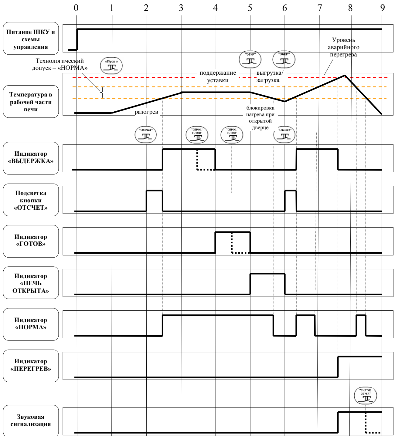
Рисунок 2 – Временные диаграммы работы шкафа.
