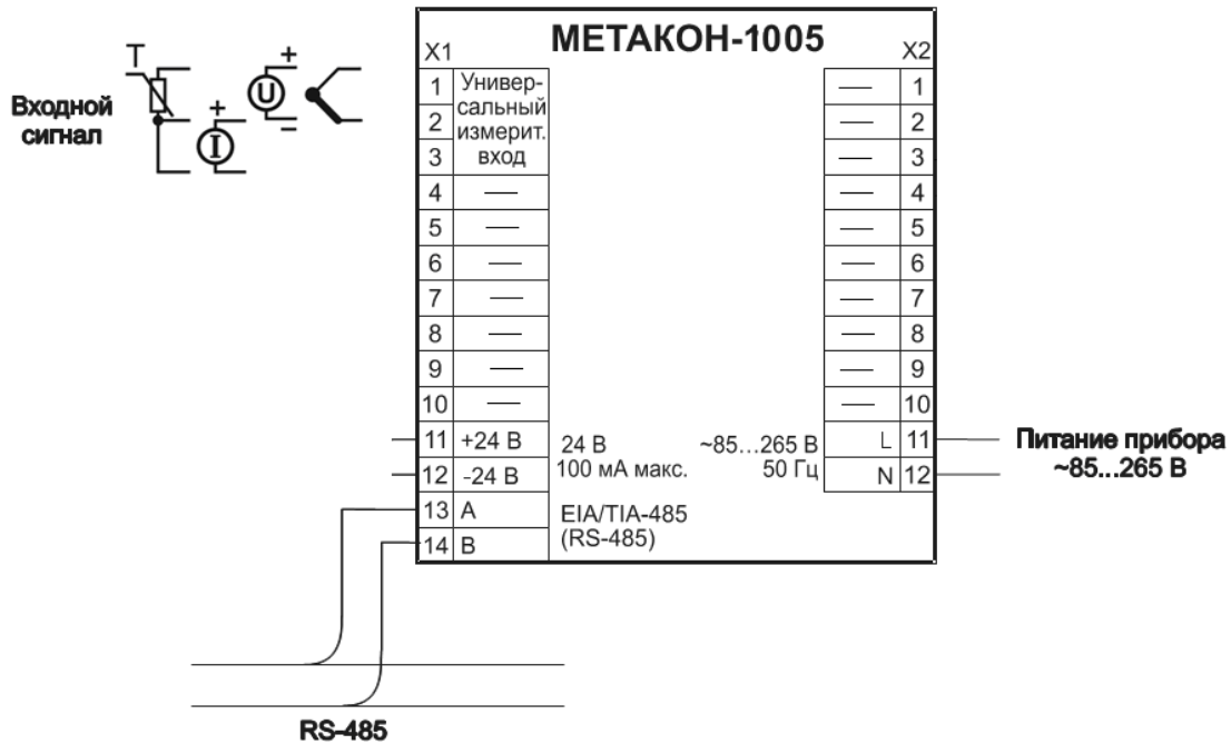
Рисунок 10 – Электрическая схема подключения прибора METAKON-1005
