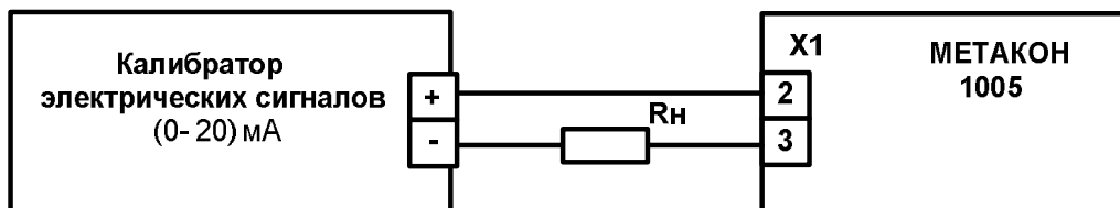
Рисунок А.6.3.1.2 – Схема подключения прибора МЕТАКОН-1005 для проведения проверки по сигналам тока
